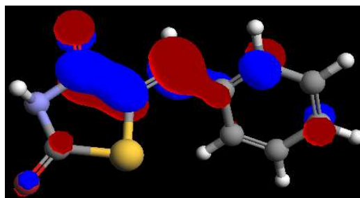
LUMO of 1a
