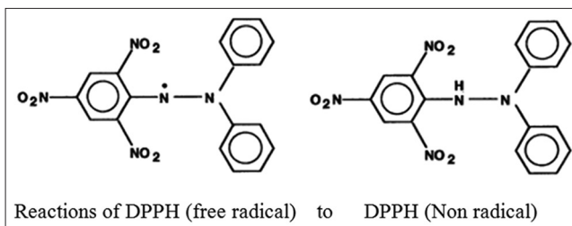
Fig. 6: 1, 1-diphenyl-2-picrylhydrazyl
