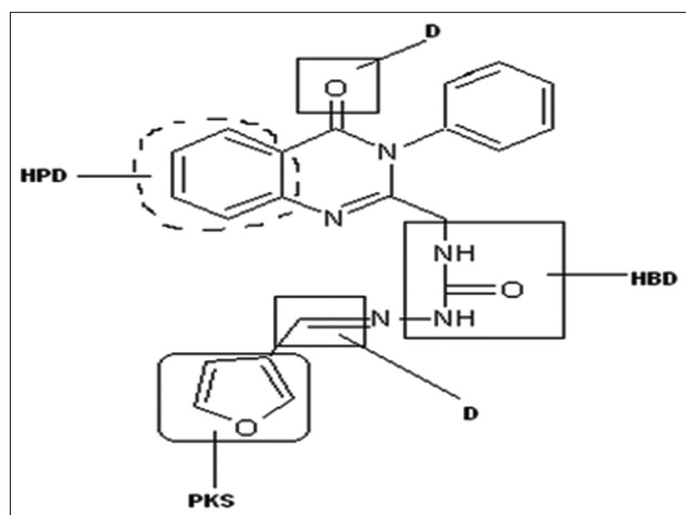
Fig. 1: Quinazolinone pharmacophore
